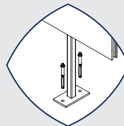
Freistehend (Verschraubung)
